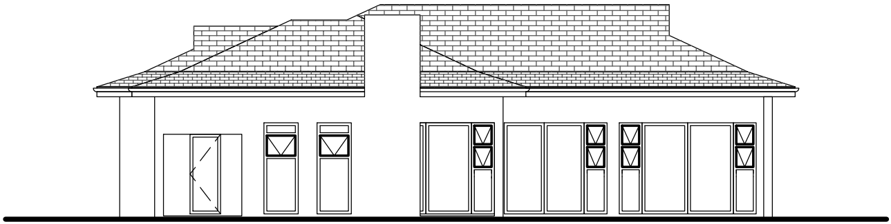
ELEVATION
